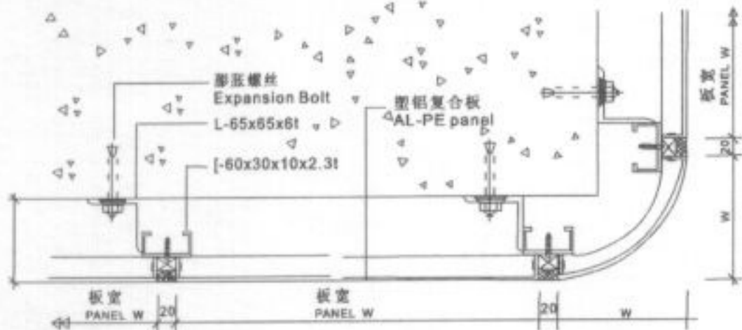
弧形转角平断面 PLAN SECTION
