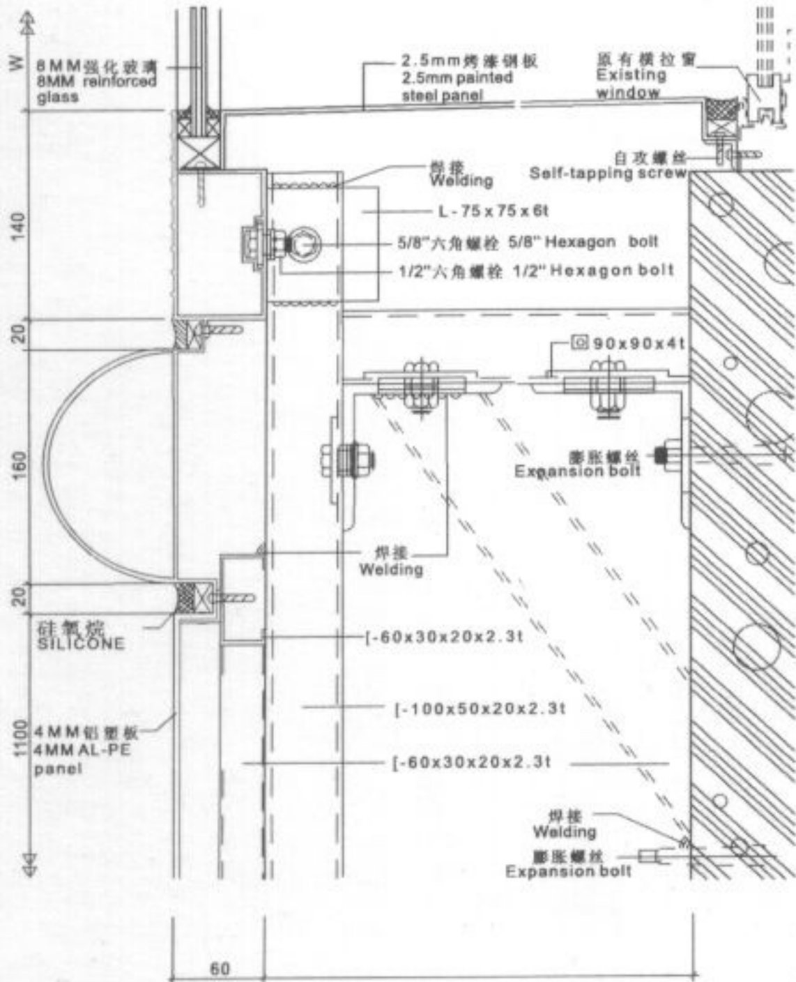
固定窗立断面图
