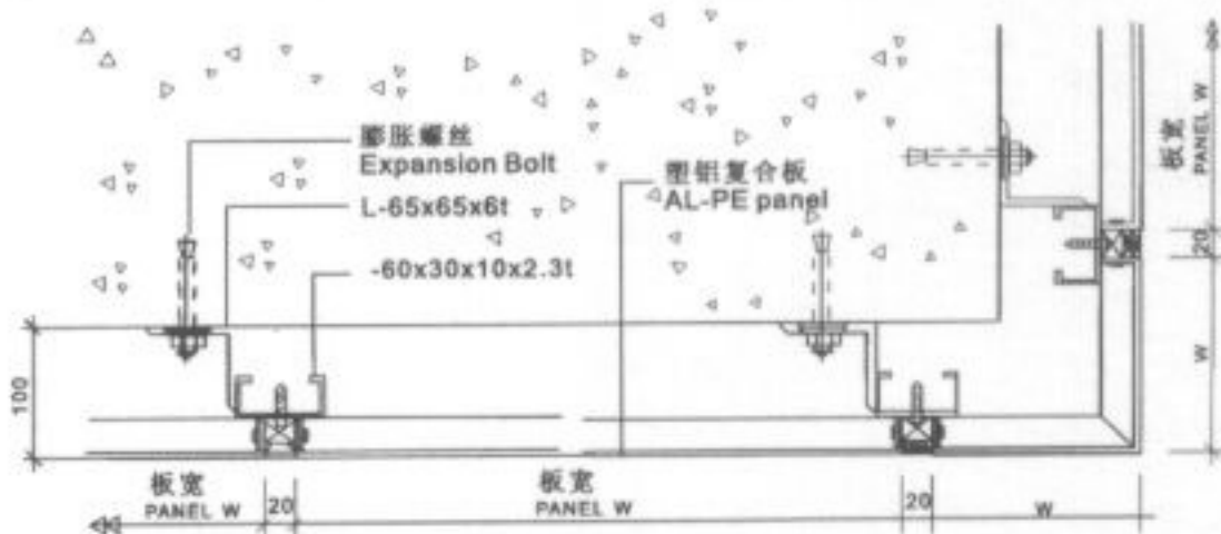
外转90° 立面图 EXTERNAL PLAN SECTION
