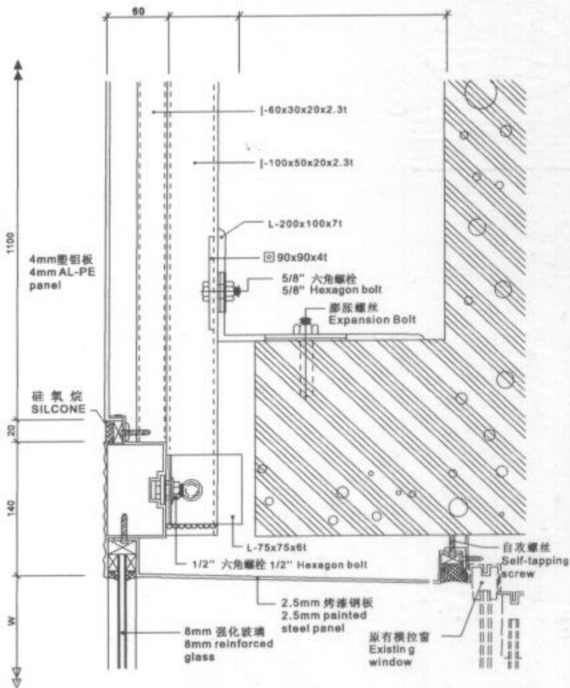
固定窗立断面图 Fixed window vertical section
